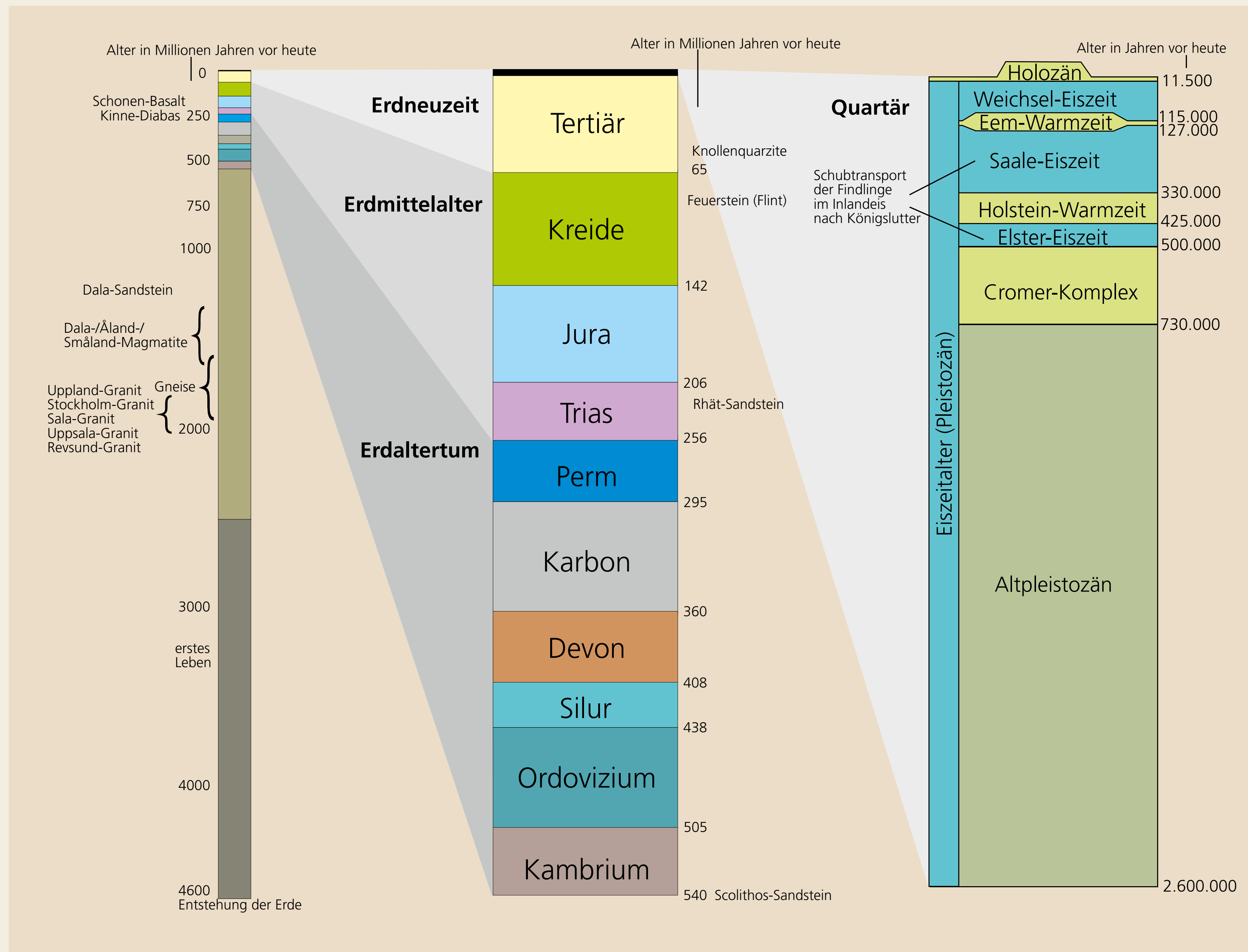
Erdgeschichtliche Übersichtstabelle mit Zuordnung der Entstehungszeit von hier aufgestellten Findlingen, die wichtige Leitgeschiebe oder Lokalgeschiebe sind. Auch sind die eiszeitlichen Schubphasen verzeichnet, in denen Findlinge von Skandinavien nach Ostfalen verfrachtet wurden.
