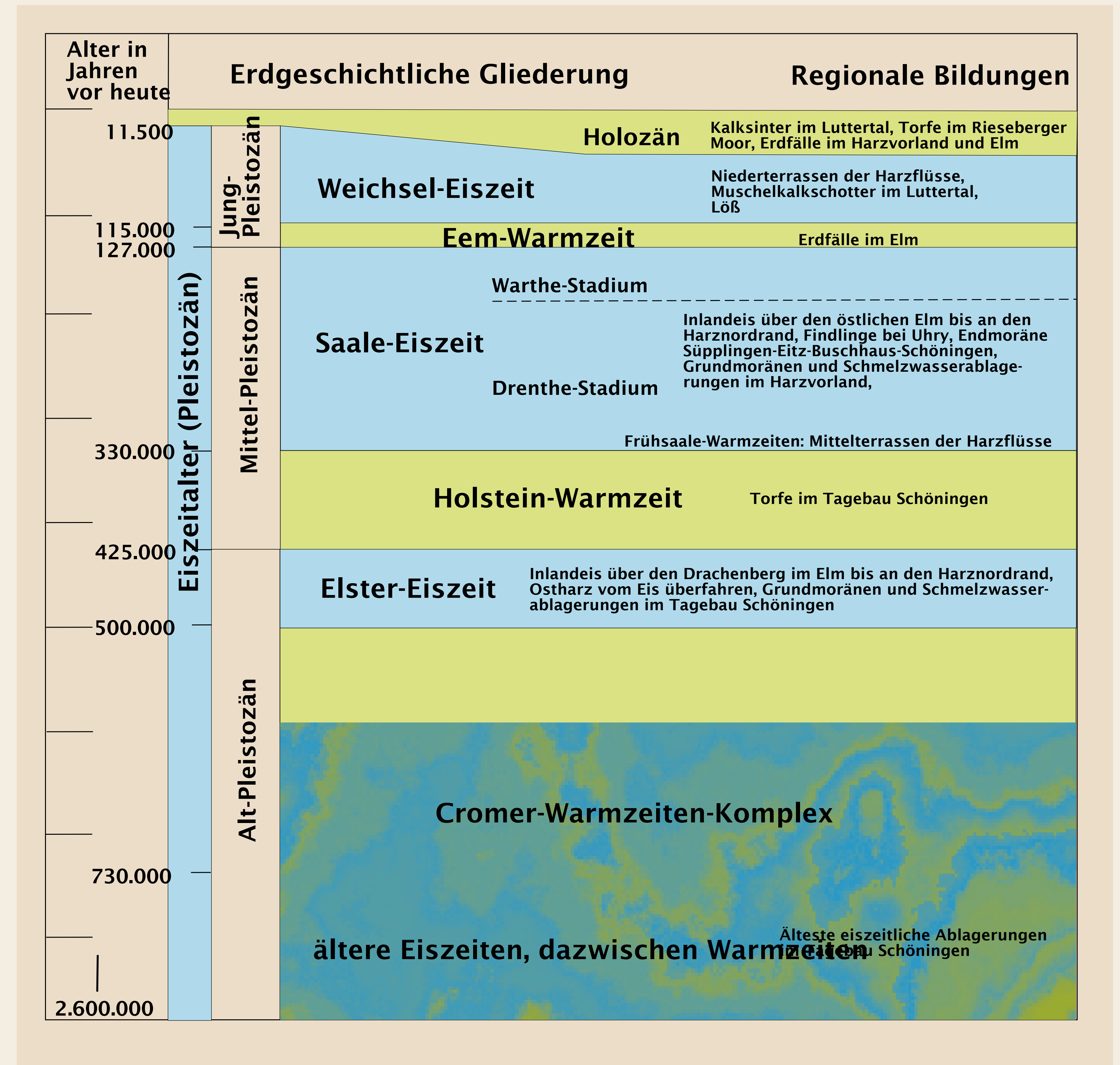
Gliederung des Quartärs im Braunschweiger Land mit der Zuordnung regional geologischer Bildungen.
